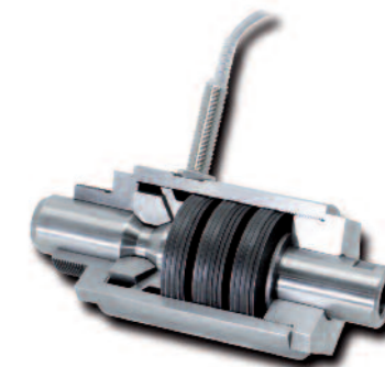
力限制器 用作连杆过载保护装置
