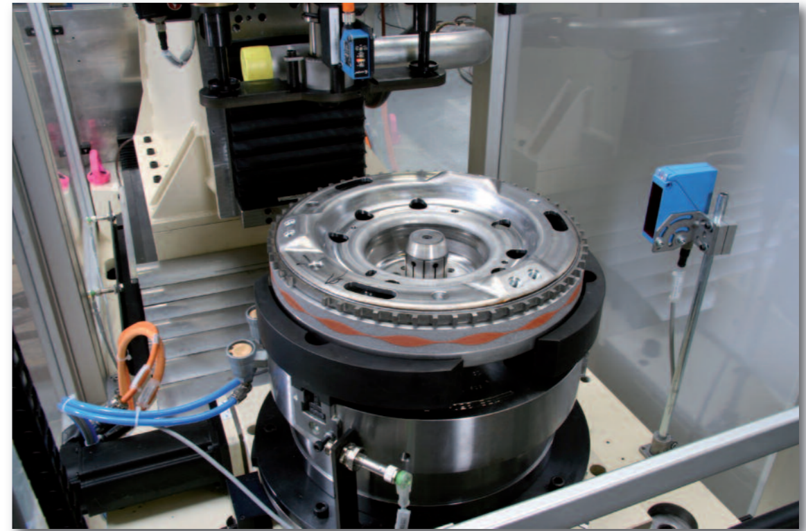
动平衡
